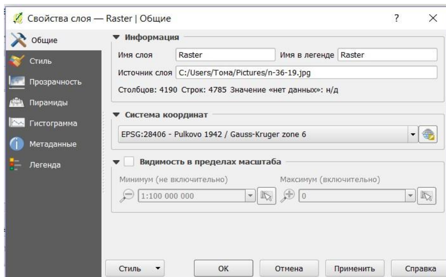
Рис. 3. Вкладка «Общие» в свойствах слоя
